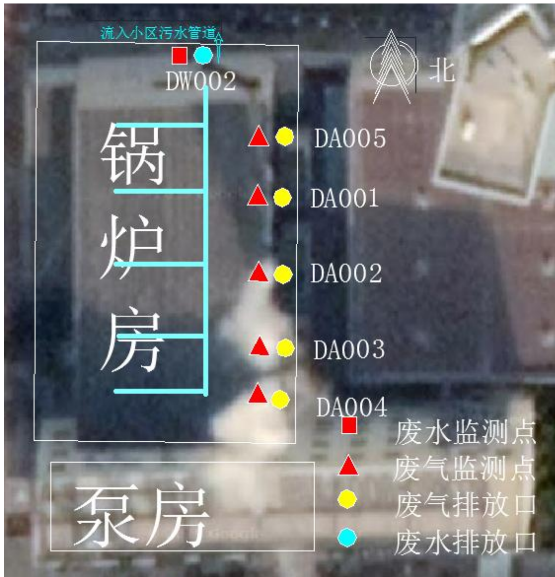
图 1 监测点位图
