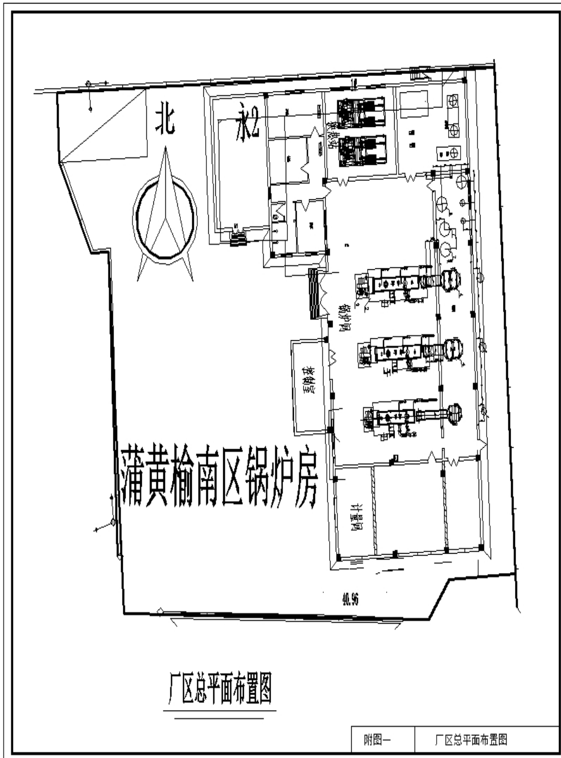
附件 3：厂区总平面布置图
